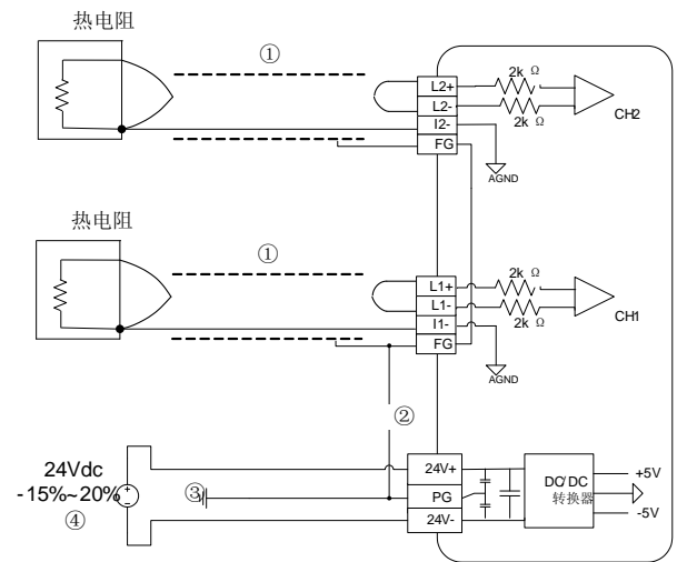
图 2-5 MC200-2PT 用户端子布线示意图
