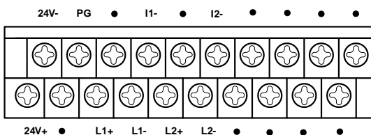
图 4-1 MC200-2PT 热电阻模块用户端子图
